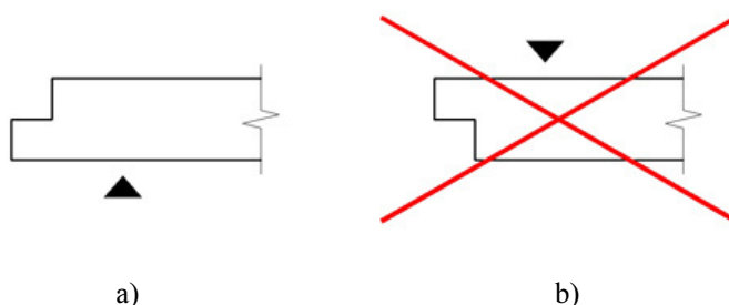
1. attēls. Veidņu virsmas apzīmējuma pielikšanas vieta
